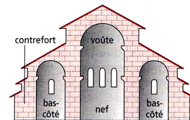
2 Coupe d'une église romane
