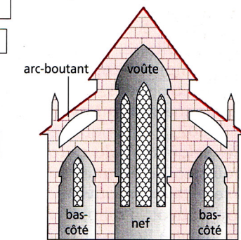
3 Coupe d'une église gothique
